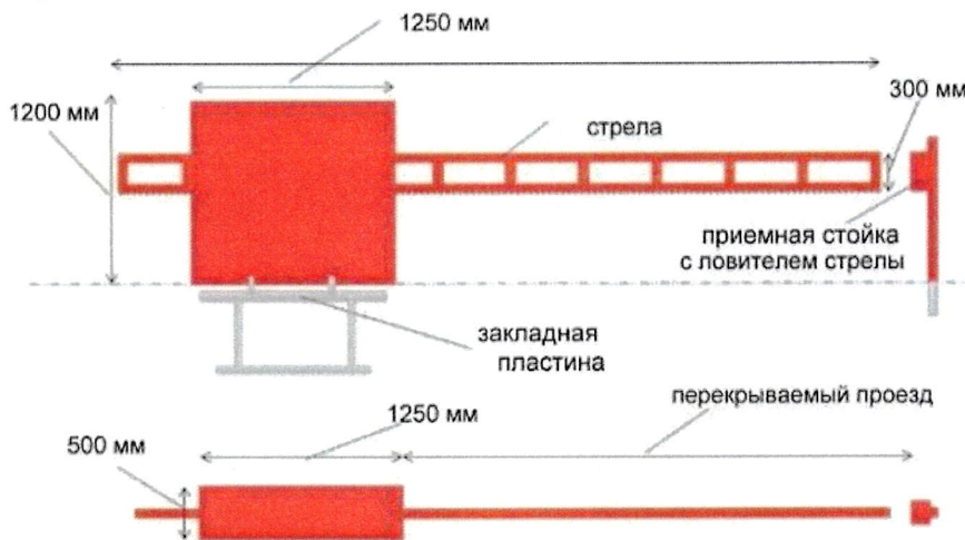
Рисунок 1 – Внешний вид и приблизительные габариты ОУ
